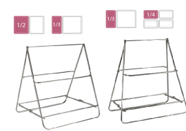
不銹鋼折疊展示架 A小姐 SIZE 10" 360x200x386mm SKU 903110 14" 355x305x375mm SKU 903114 顏色: 銀色 (ss)
